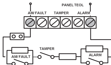
Diagrama Esquemático das Resistências EOL
