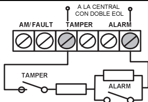
Esquema de conexión de las resistencias de final de línea
