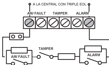
Esquema de conexión de las resistencias de final de línea
